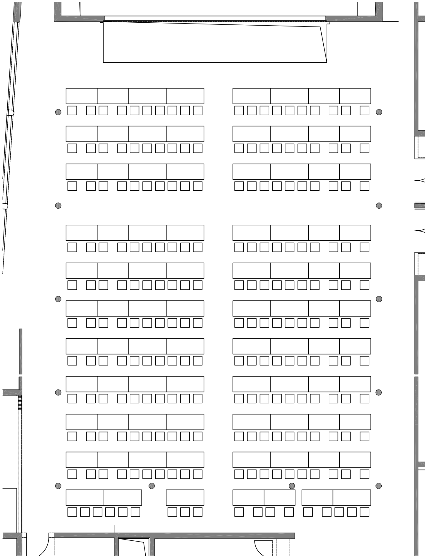
Plan Nr. 11 Parlamentarisch Großer Saal 218 Sitzplätze M1/100
